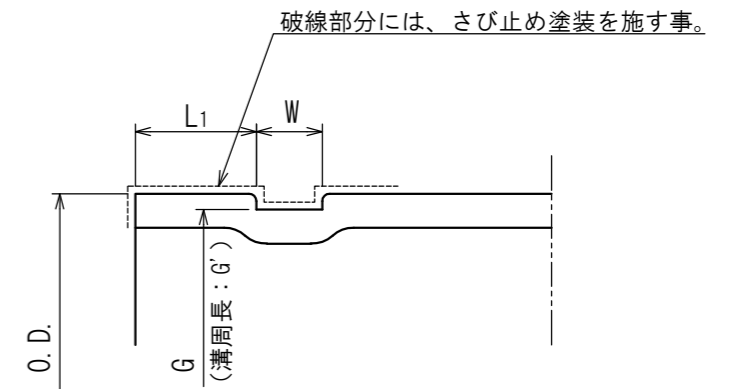
管端寸法
